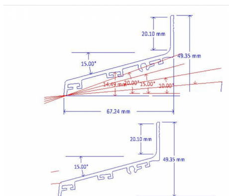
Schéma de section coté Dimensions exprimées en mm.
